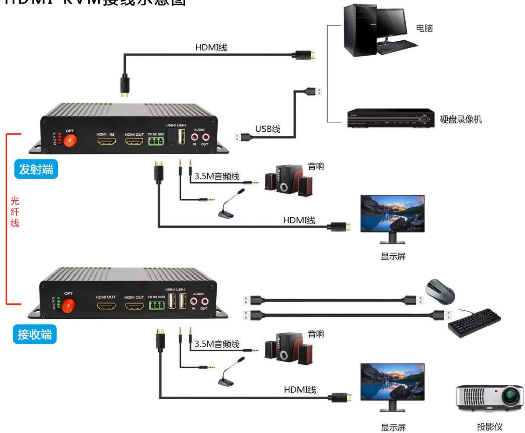
HDMI-KVM接线示意图
